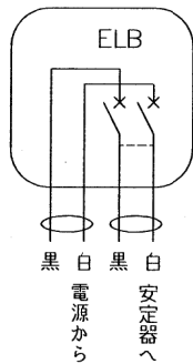
結線図
